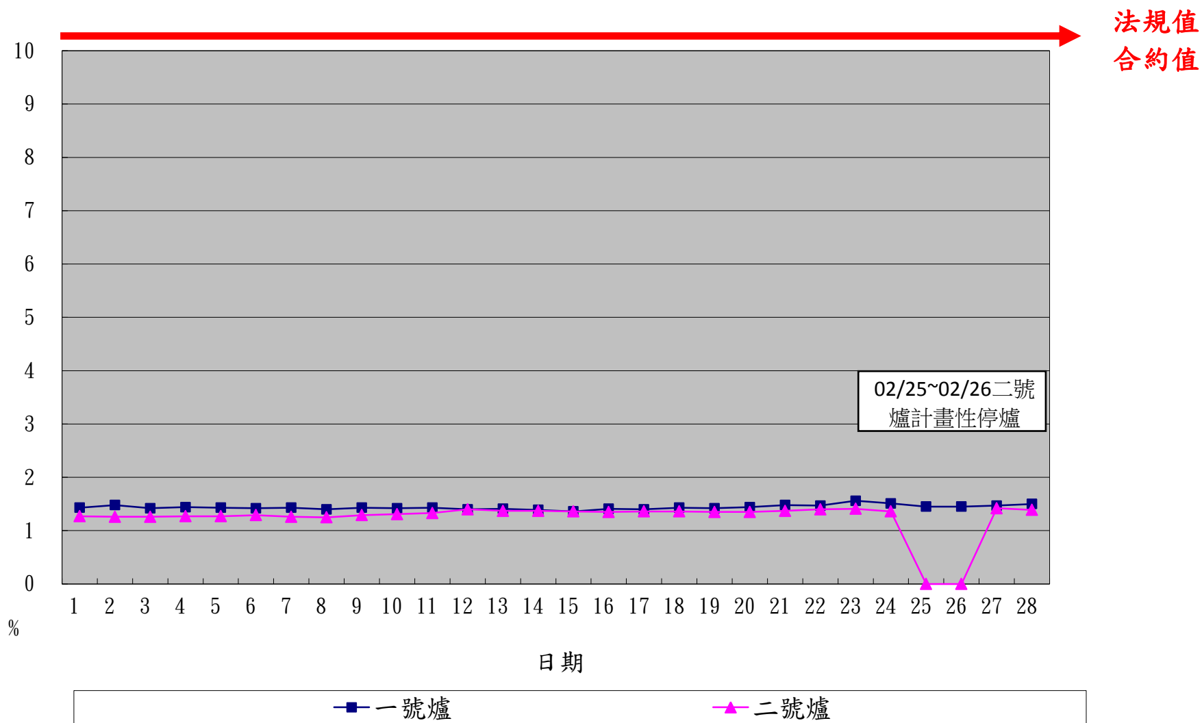
一百零六年二月份 OPACITY單日24小時整月排放監測紀錄
