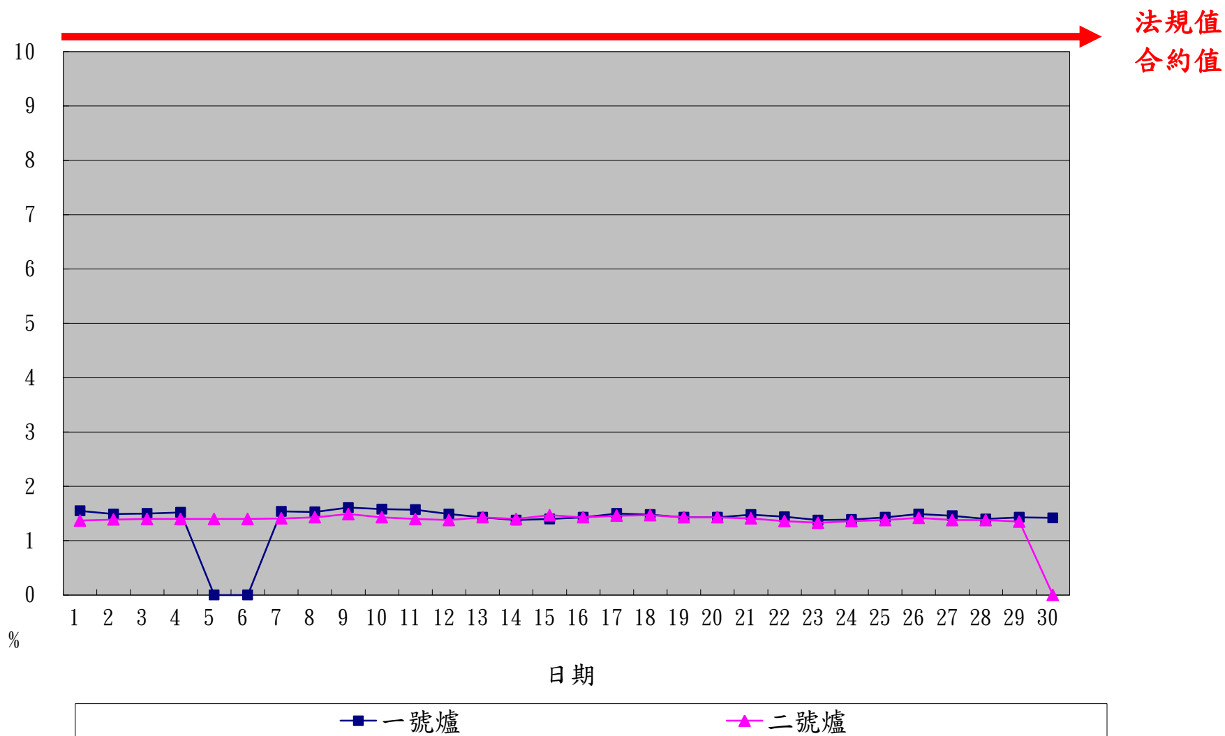
一百零六年四月份 OPACITY單日24小時整月排放監測紀錄
