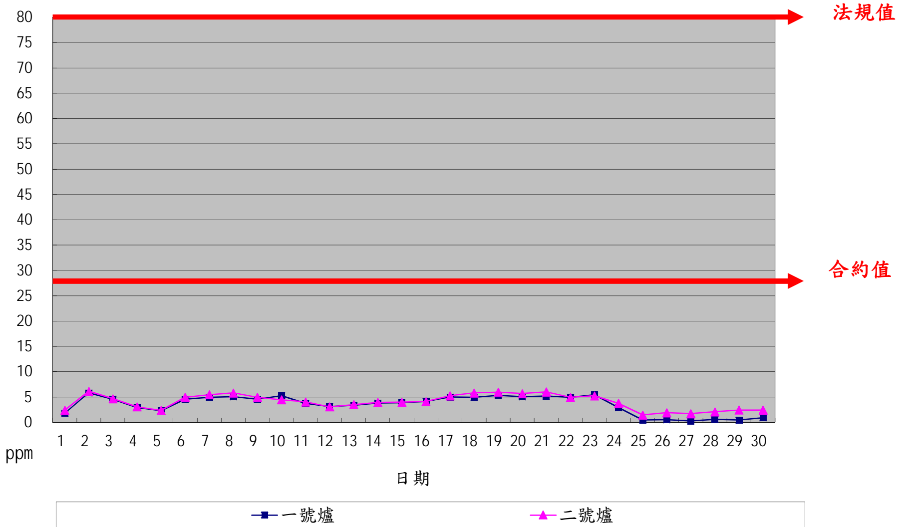
一百零四年六月份 SO x 單日24小時整月排放監測紀錄
