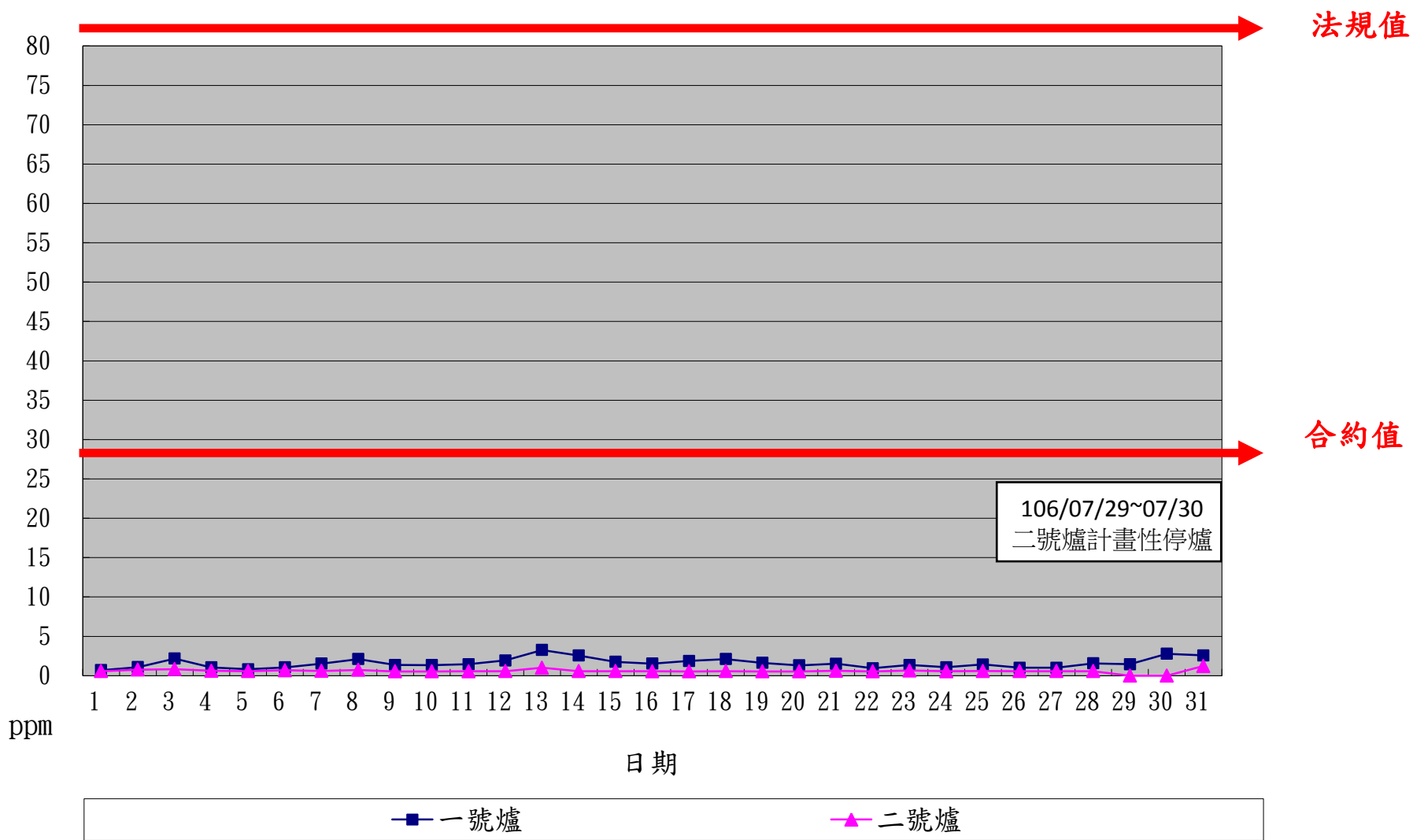
一百零六年七月份 SO x 單日24小時整月排放監測紀錄
