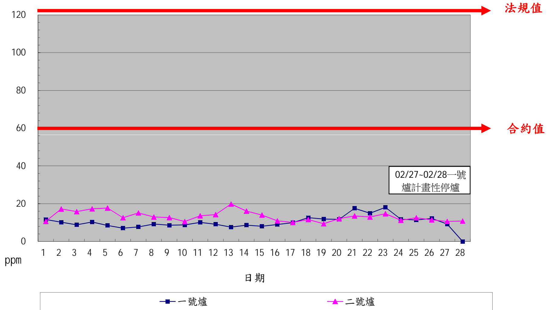
一百零三年二月份 CO 單日 24 小時平均整月排放監測紀錄
