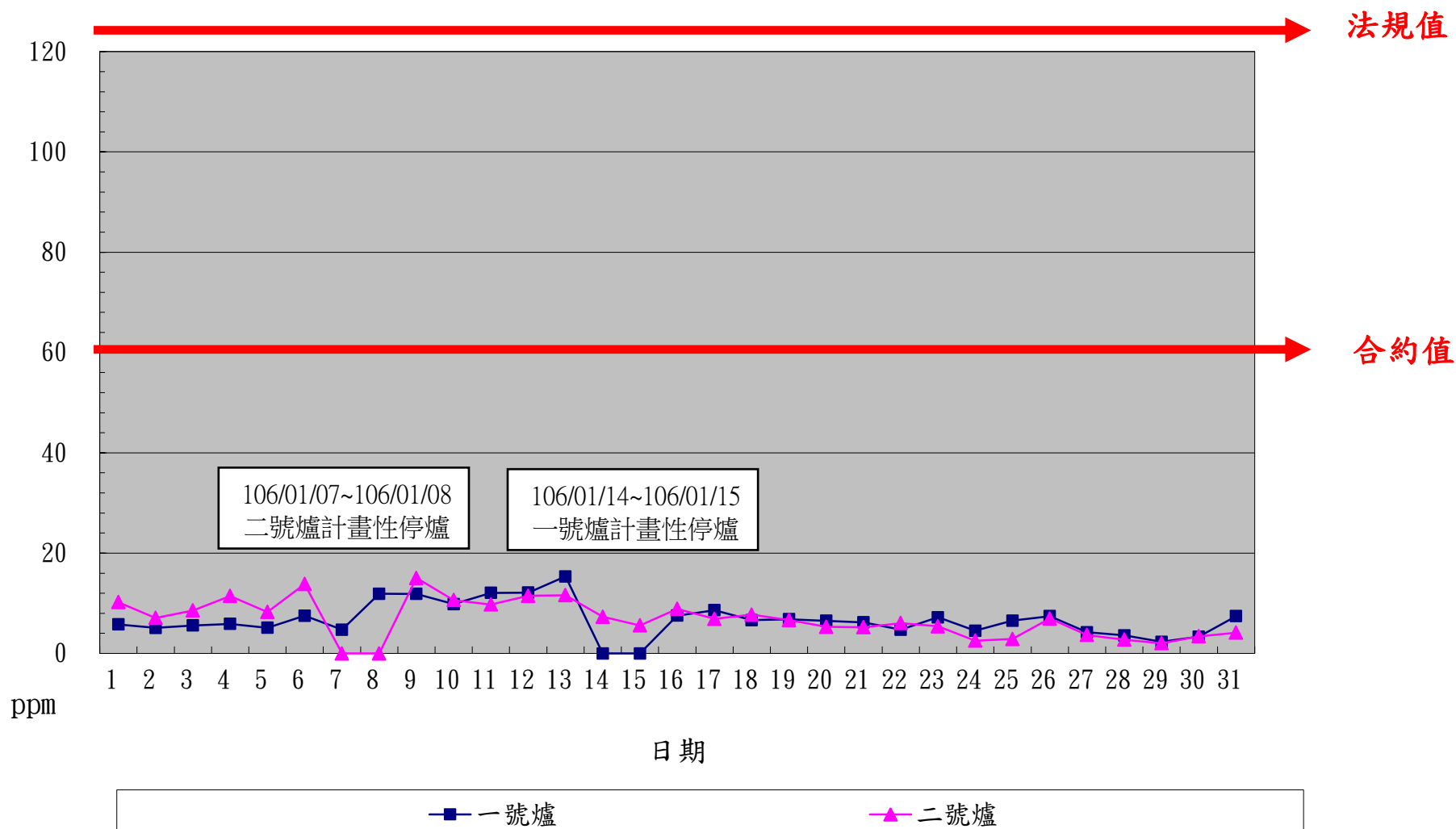
一百零六年一月份 CO 單日24小時平均整月排放監測紀錄
