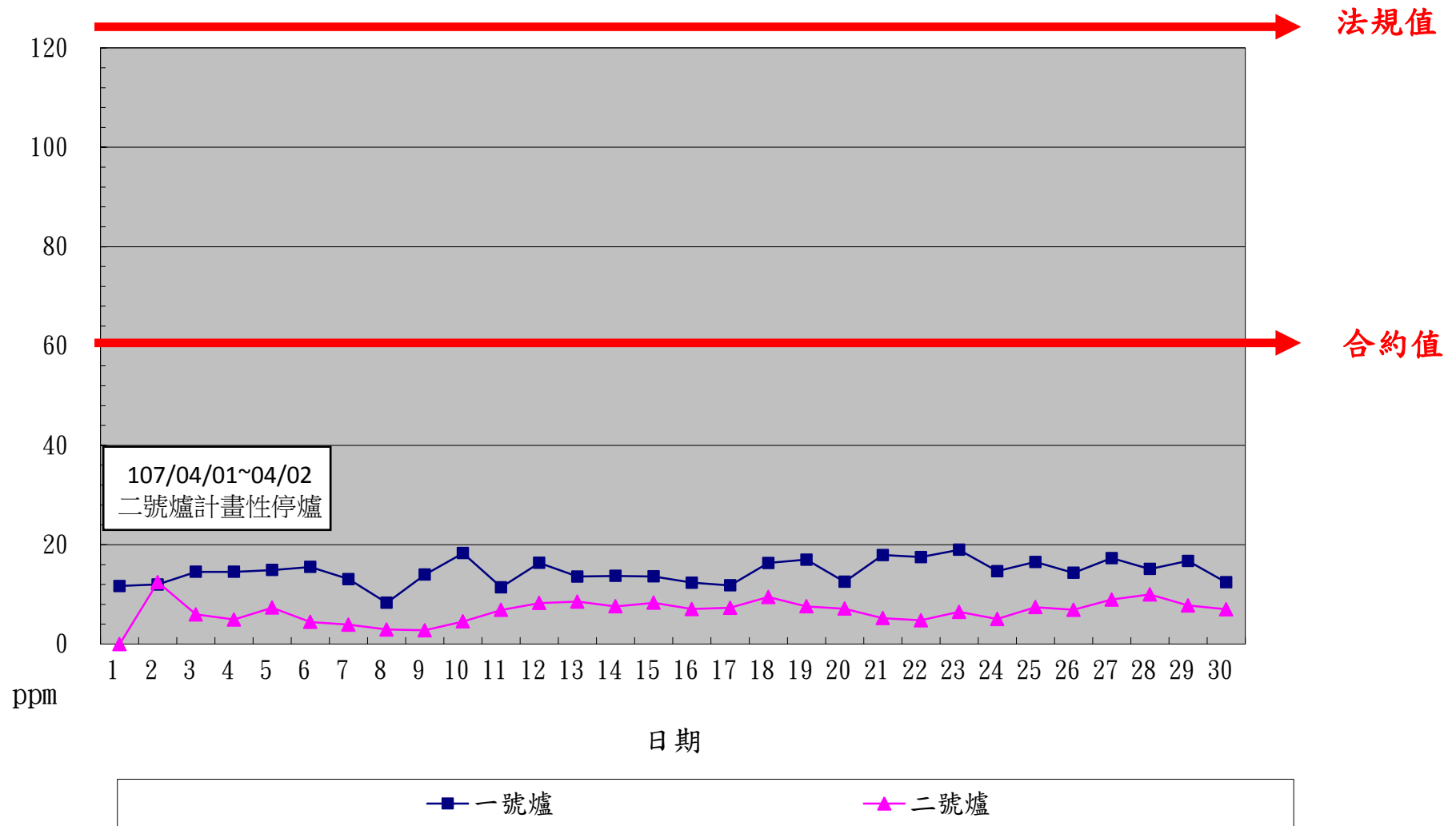
一百零七年四月份 CO 單日24小時平均整月排放監測紀錄
