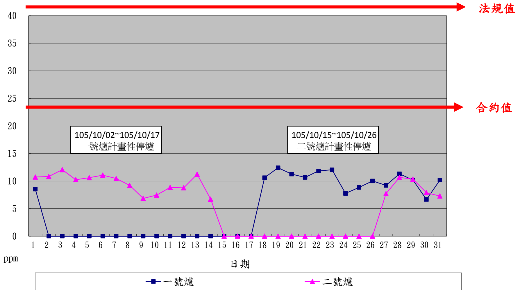
一百零五年十月份 HCl 單日24小時整月排放監測紀錄
