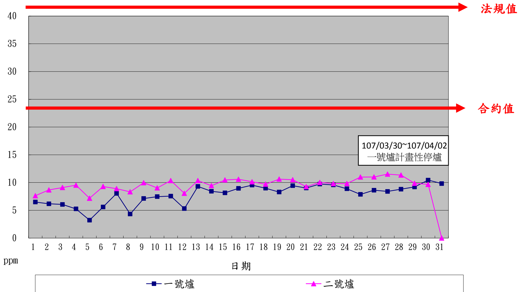
一百零七年三月份 HCl 單日24小時整月排放監測紀錄
