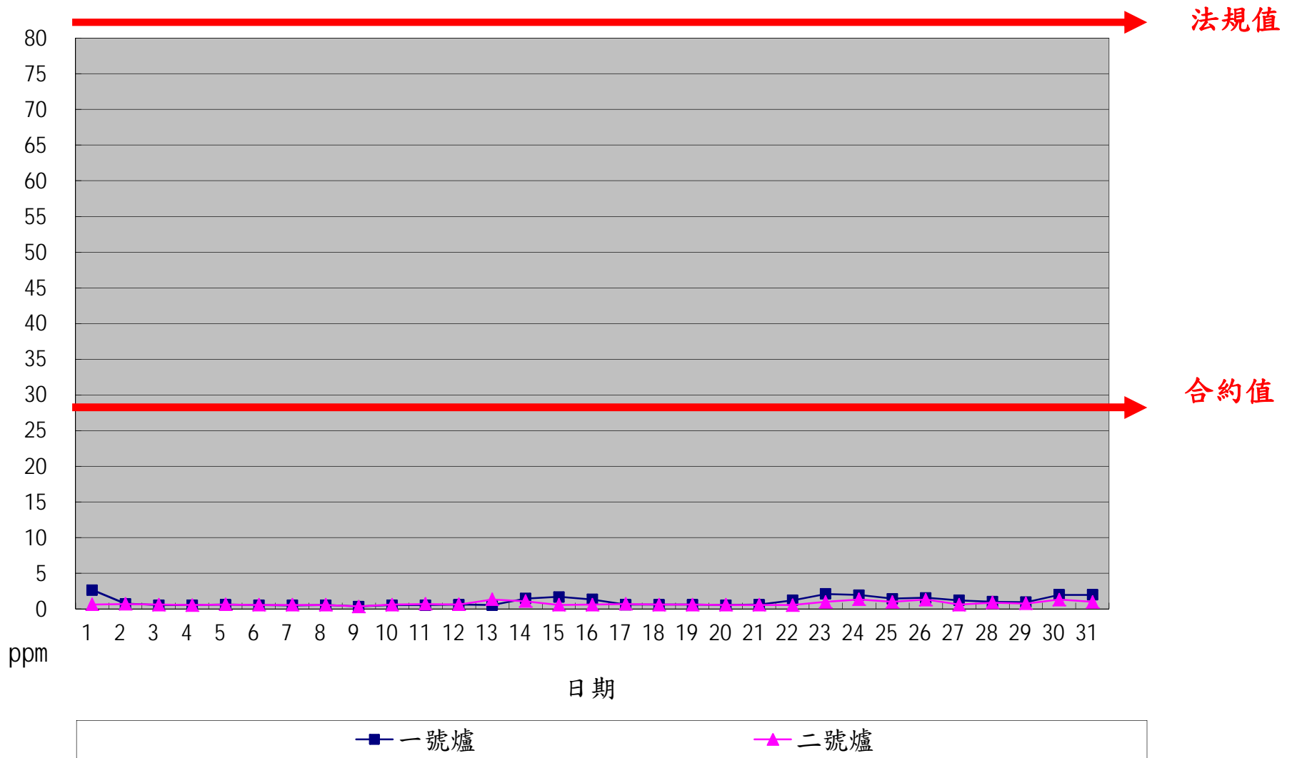
一百零七年八月份 SO x 單日24小時整月排放監測紀錄
