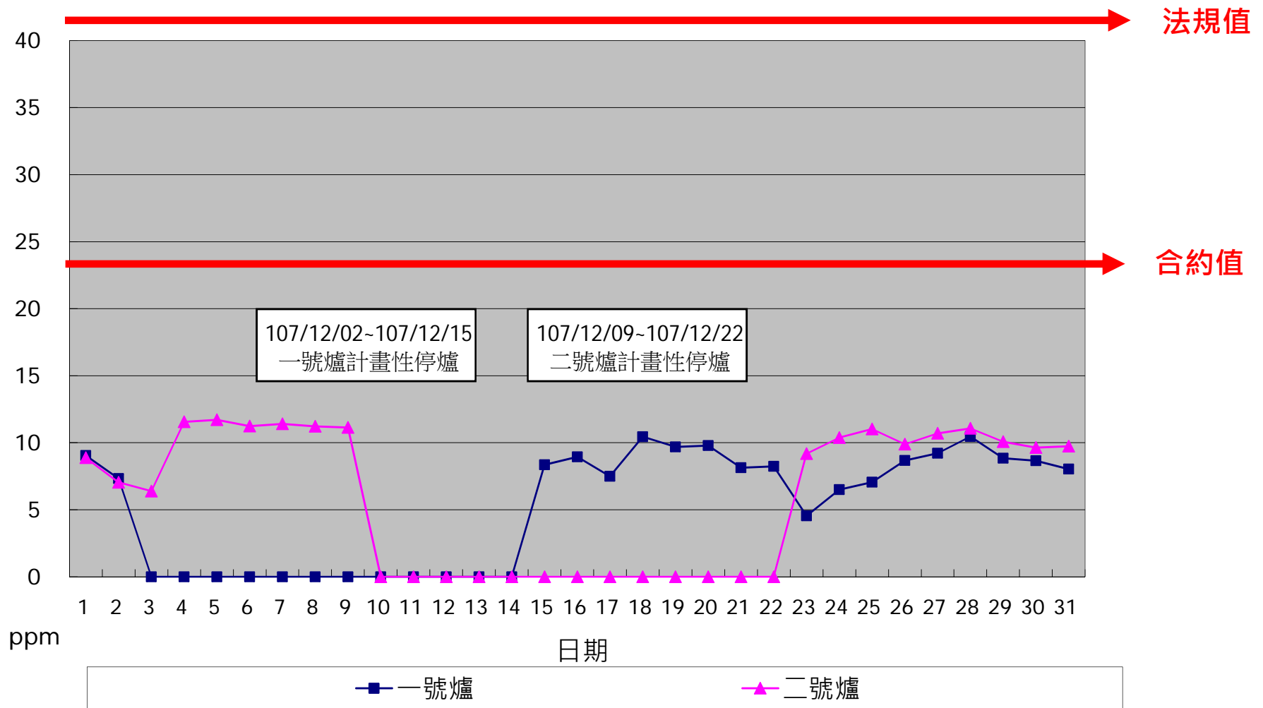
一百零七年十二月份 HCl單日24小時整月排放監測紀錄
