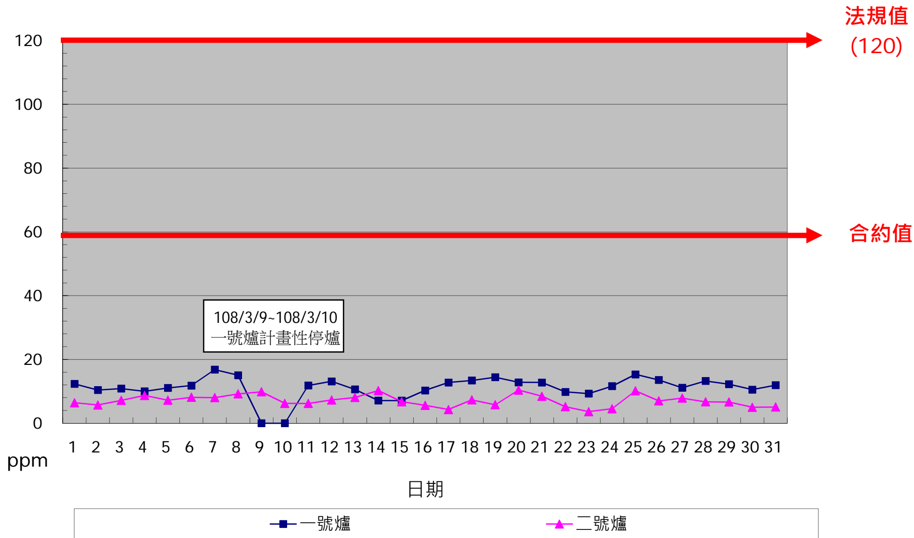
一百零八年三月份 CO 單日24小時平均整月排放監測紀錄
