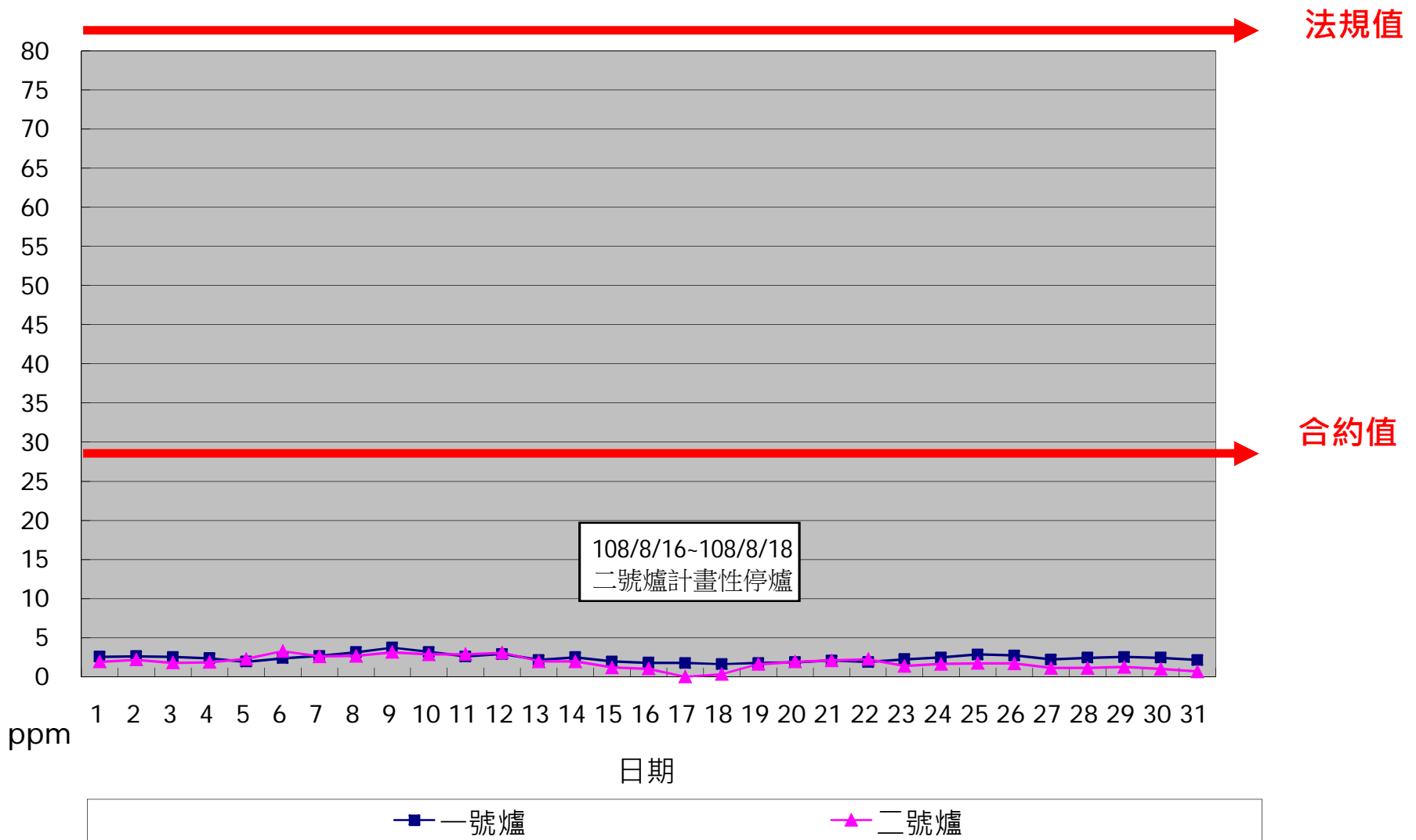
一百零八年八月份 SO x 單日24小時整月排放監測紀錄
