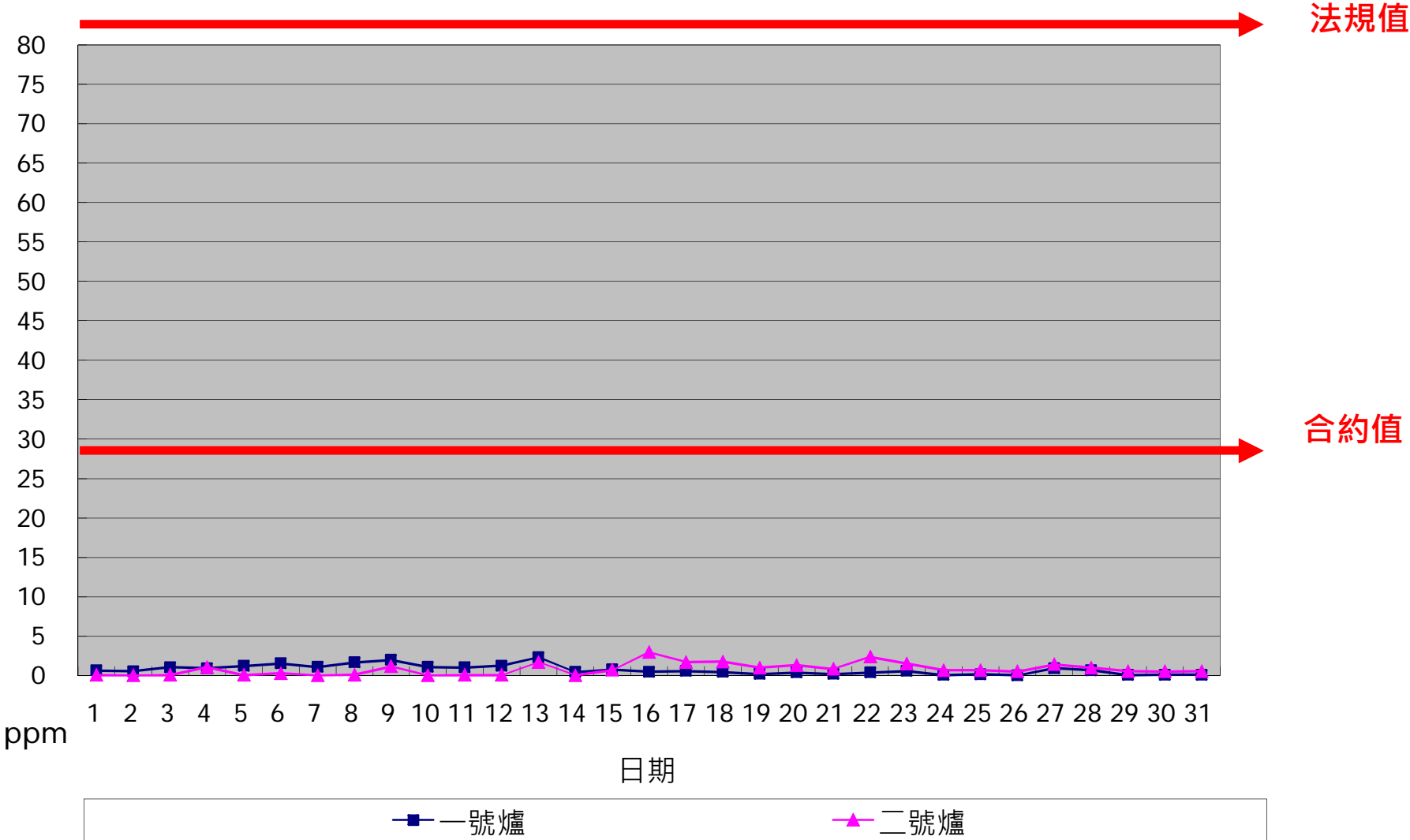
一百零九年一月份 SO x 單日24小時整月排放監測紀錄
