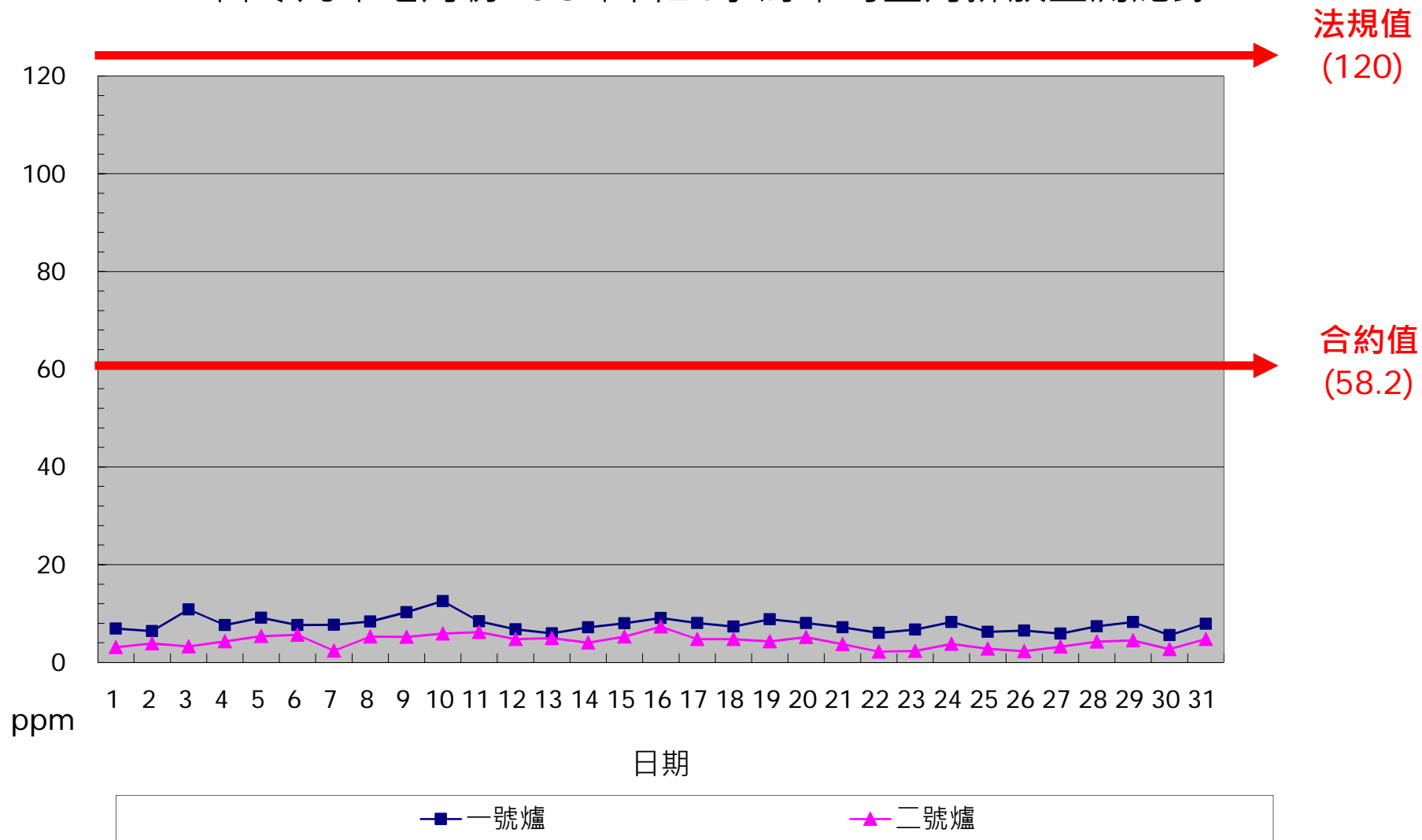
一百零九年七月份 CO單日24小時平均整月排放監測紀錄
