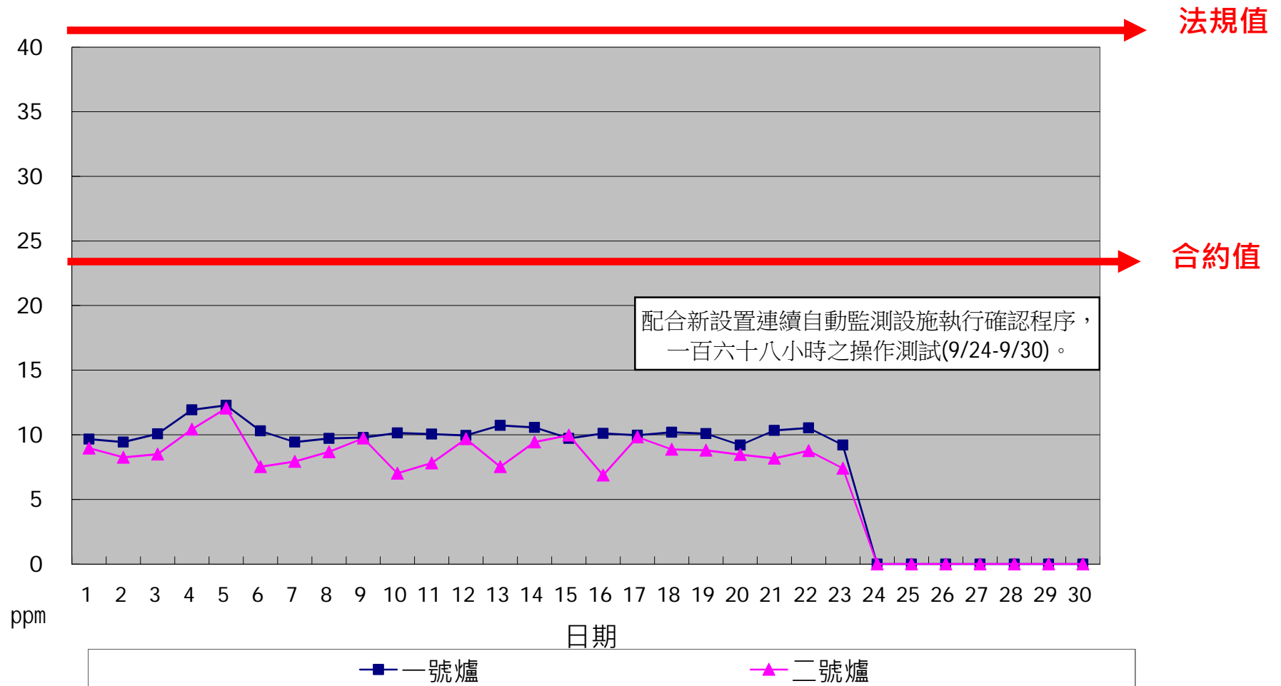
一百一十年九月份 HCl單日24小時整月排放監測紀錄
