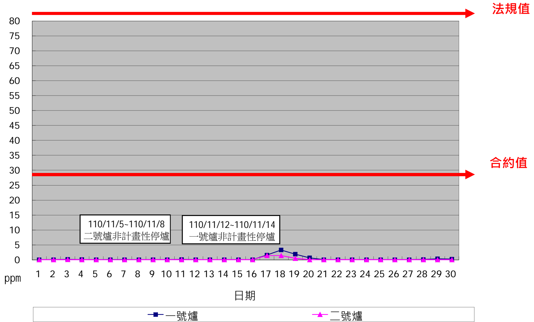
一百一十年十一月份 SO x 單日24小時整月排放監測紀錄
