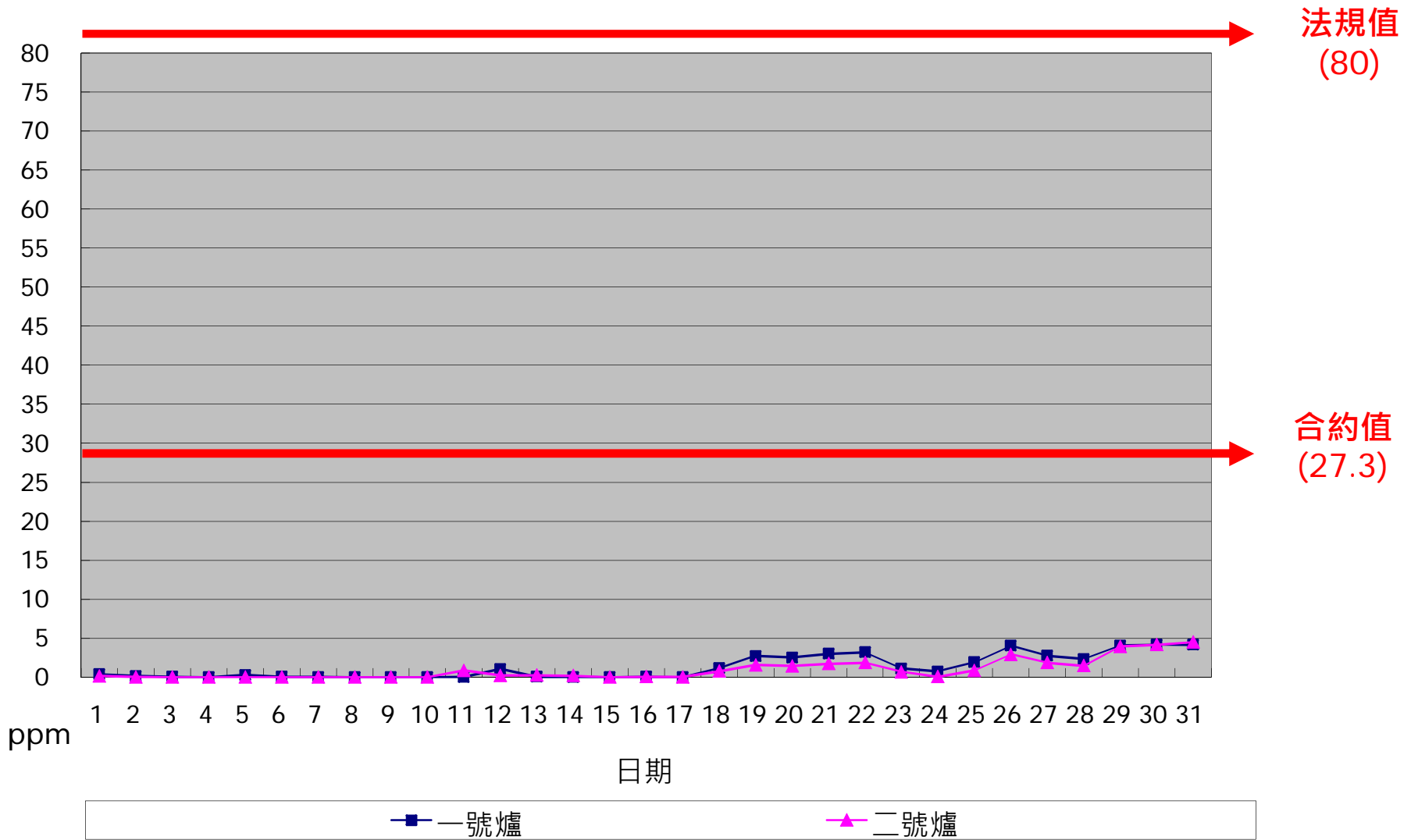
一百一十一年一月份 SO x 單日24小時整月排放監測紀錄
