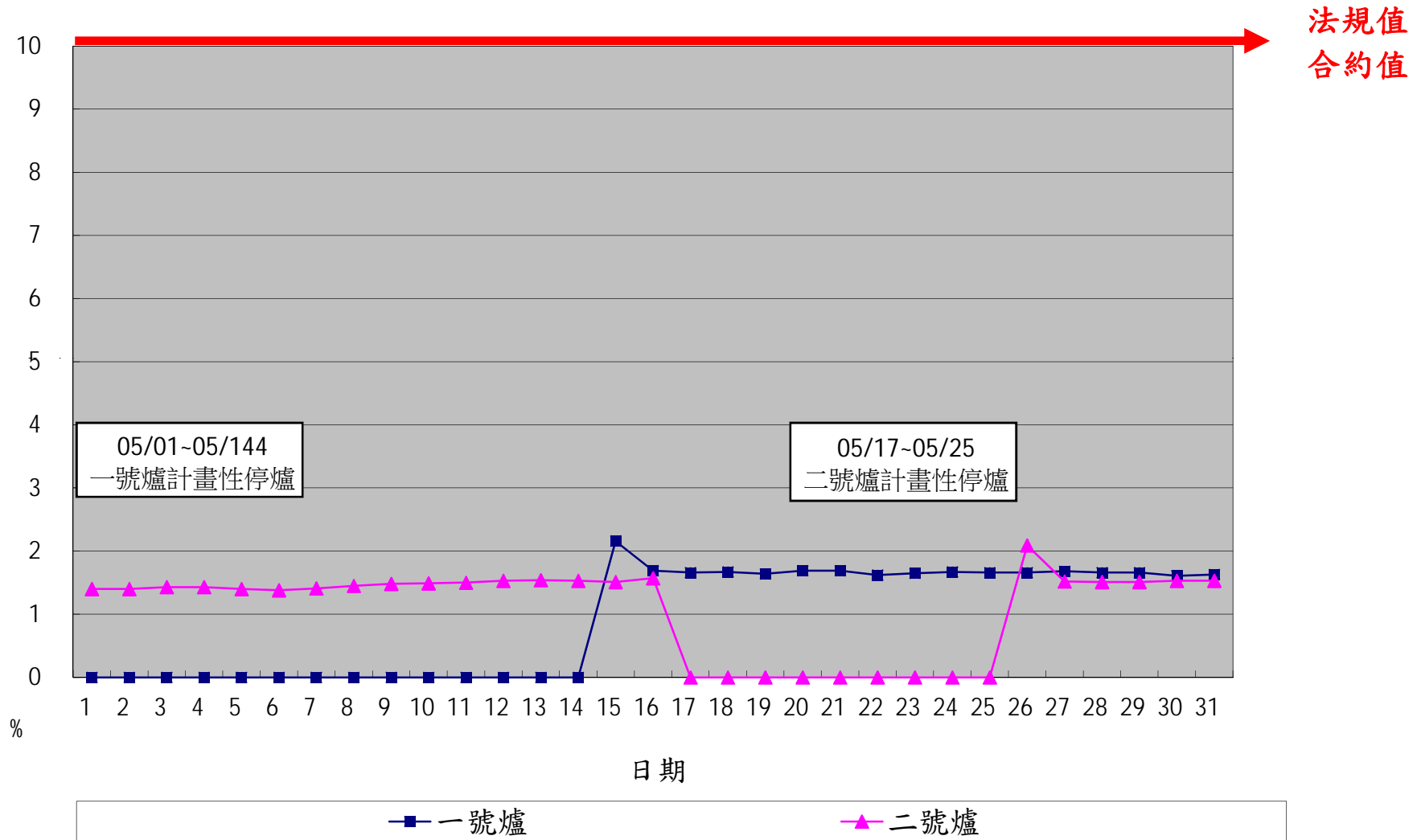
一百零三年五月份 OPACITY 單日24小時整月排放監測紀錄
