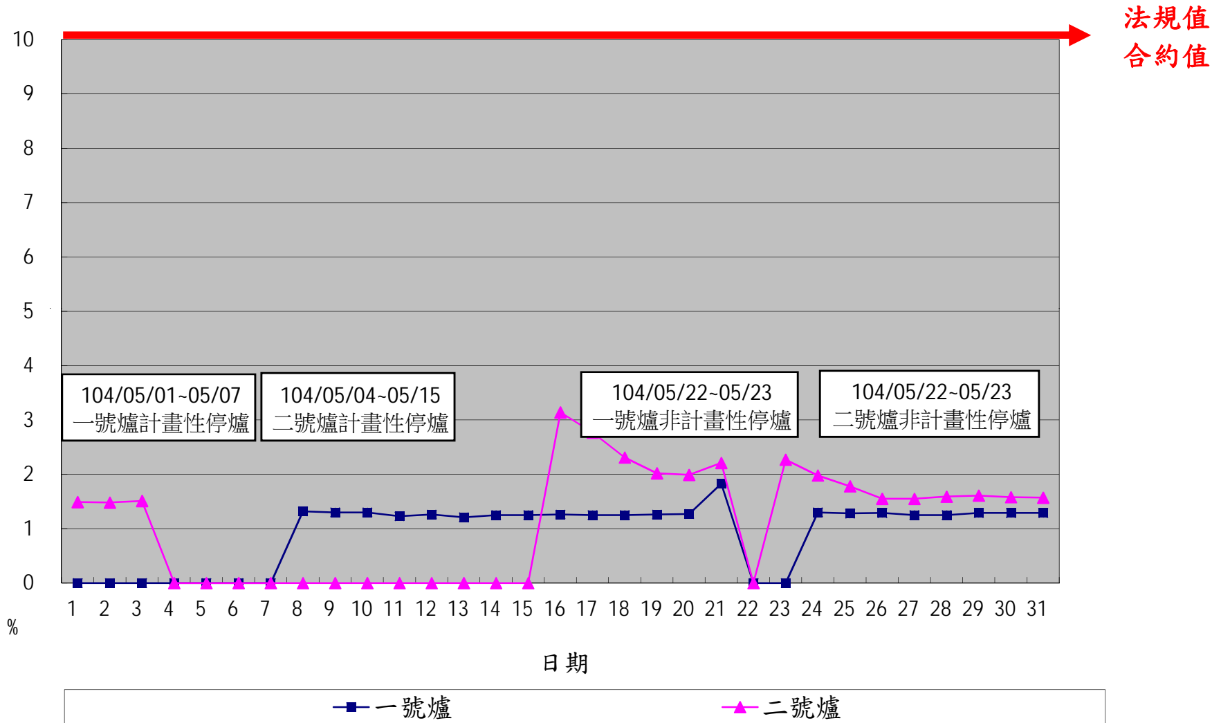
一百零四年五月份 OPACITY 單日24小時整月排放監測紀錄
