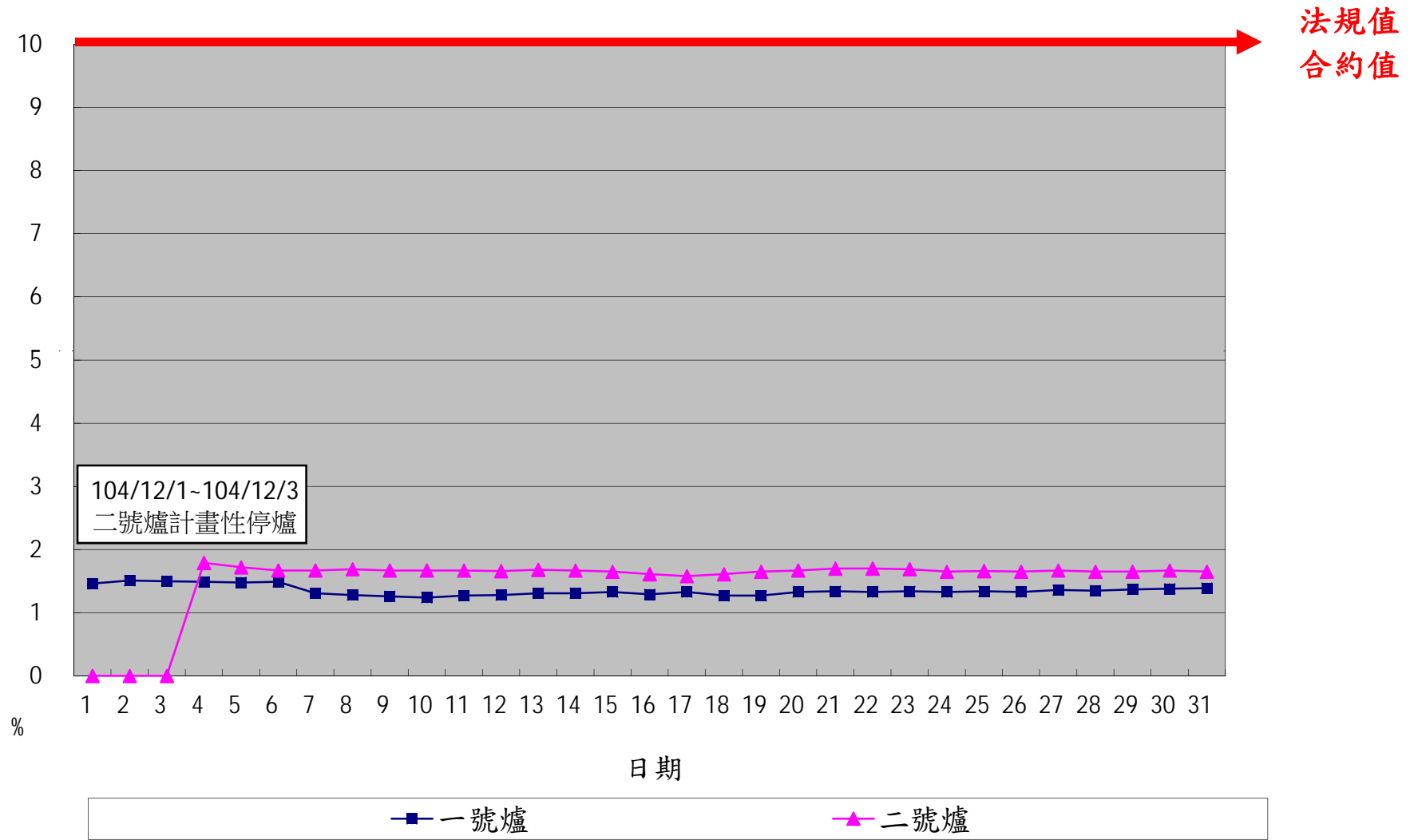
一百零四年十二月份 OPACITY單日24小時整月排放監測紀錄
