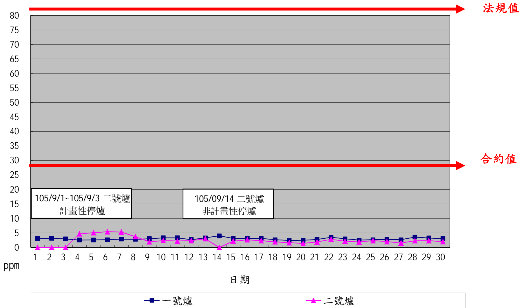
一百零五年九月份 SO x 單日24小時整月排放監測紀錄
