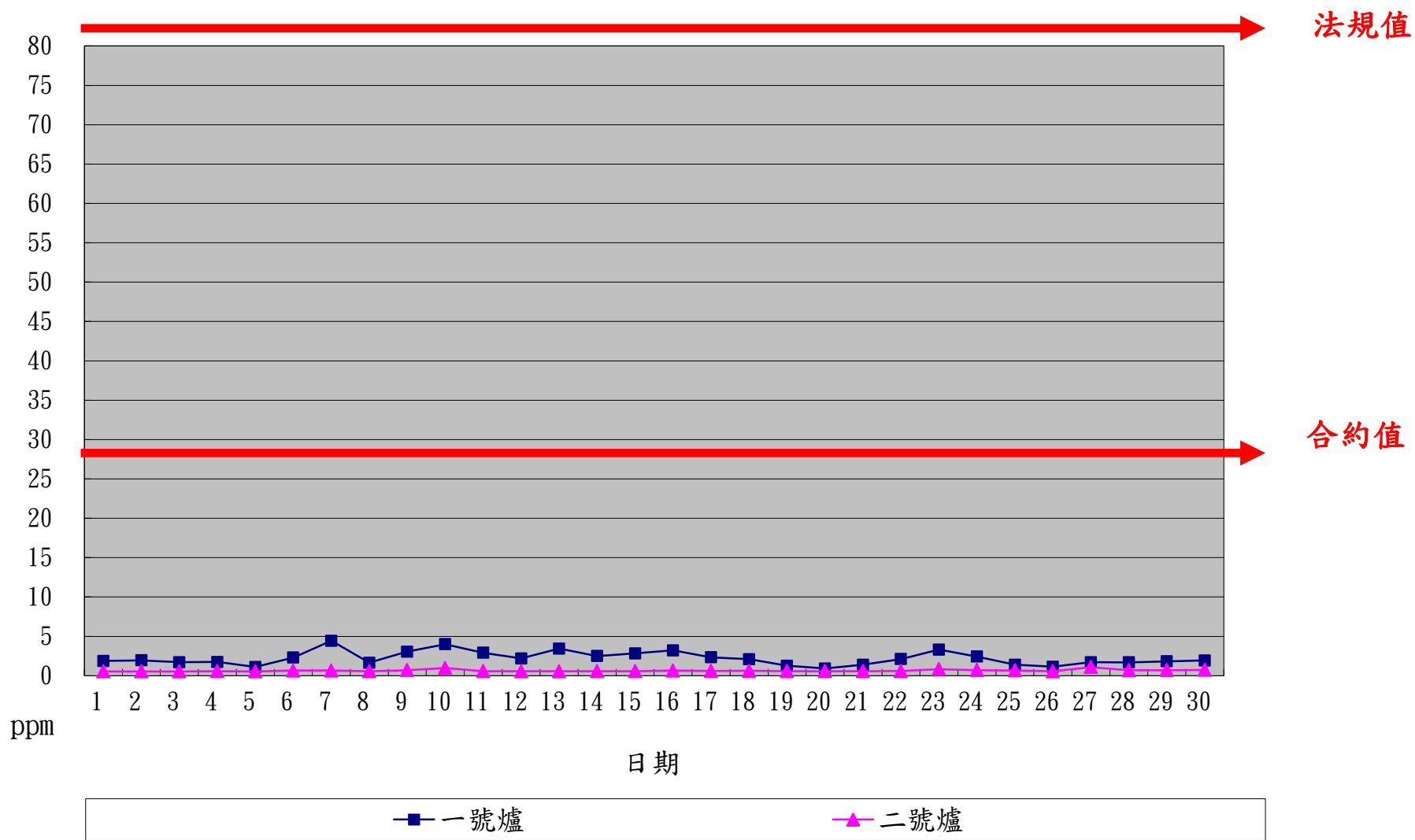
一百零六年九月份 SO x 單日24小時整月排放監測紀錄
