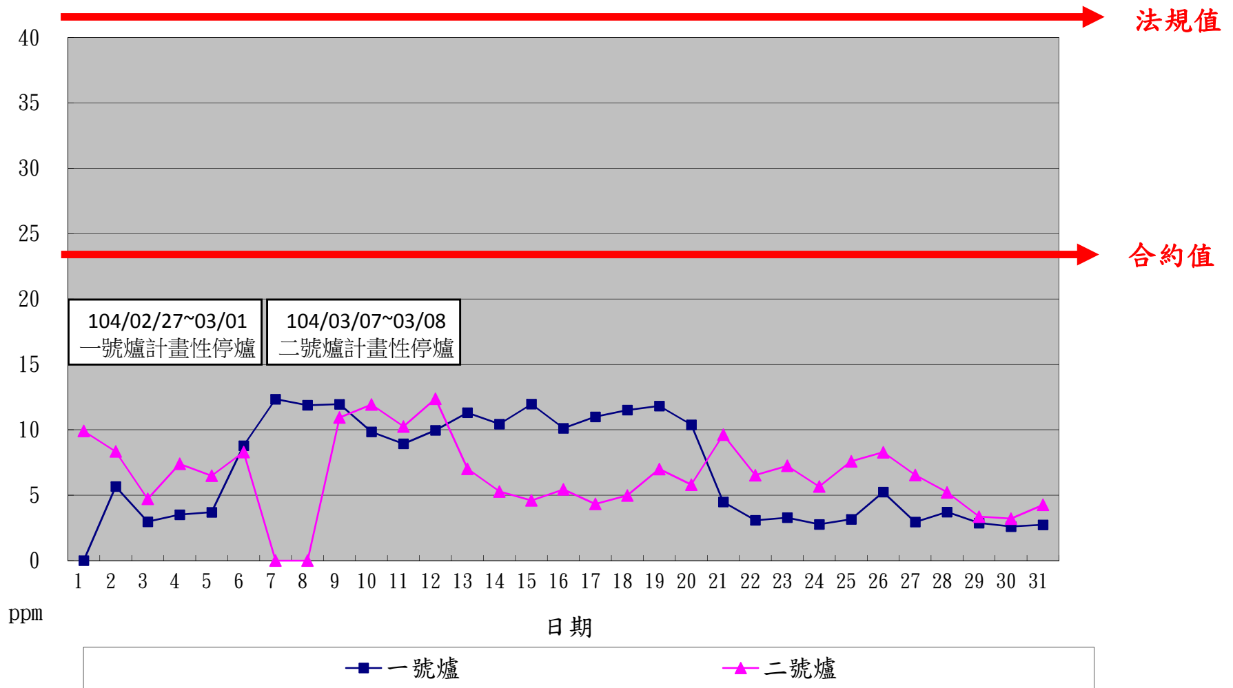
一百零四年三月份 HCl 單日24小時整月排放監測紀錄
