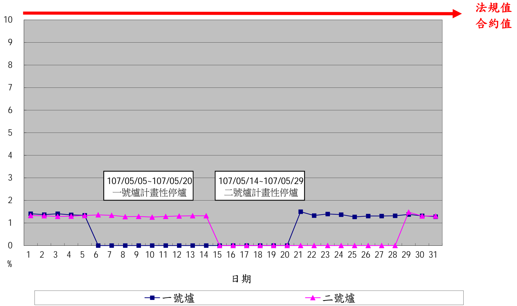
一百零七年五月份 OPACITY 單日24小時整月排放監測紀錄
