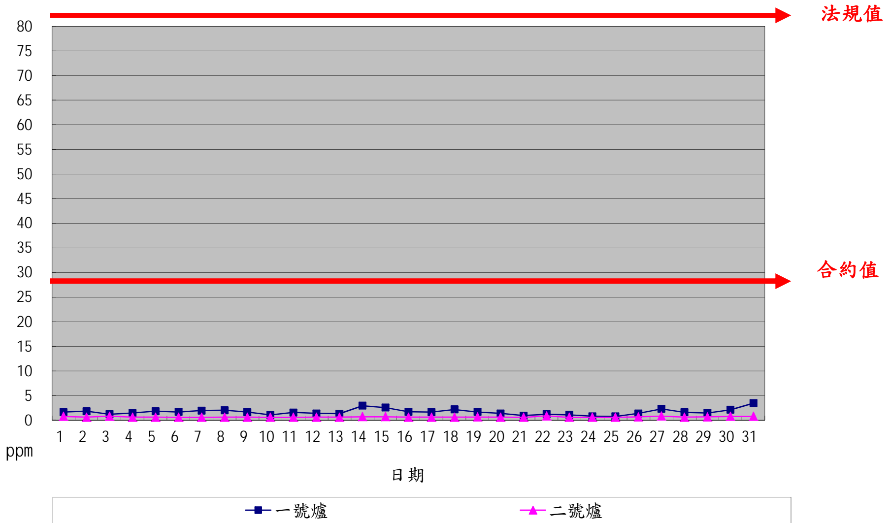
一百零七年七月份 SO x 單日24小時整月排放監測紀錄
