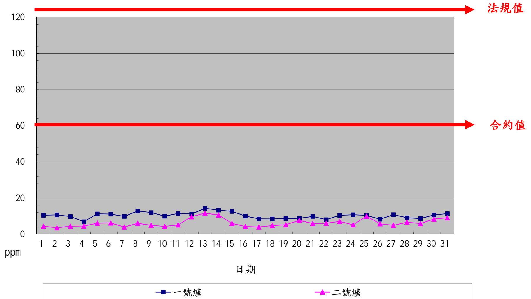
一百零七年七月份 CO 單日24小時平均整月排放監測紀錄
