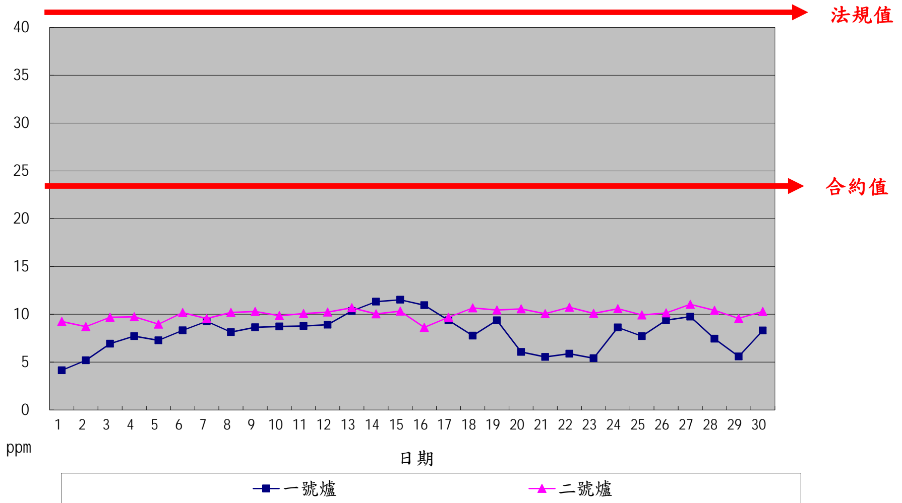
一百零八年四月份 HCl 單日24小時整月排放監測紀錄
