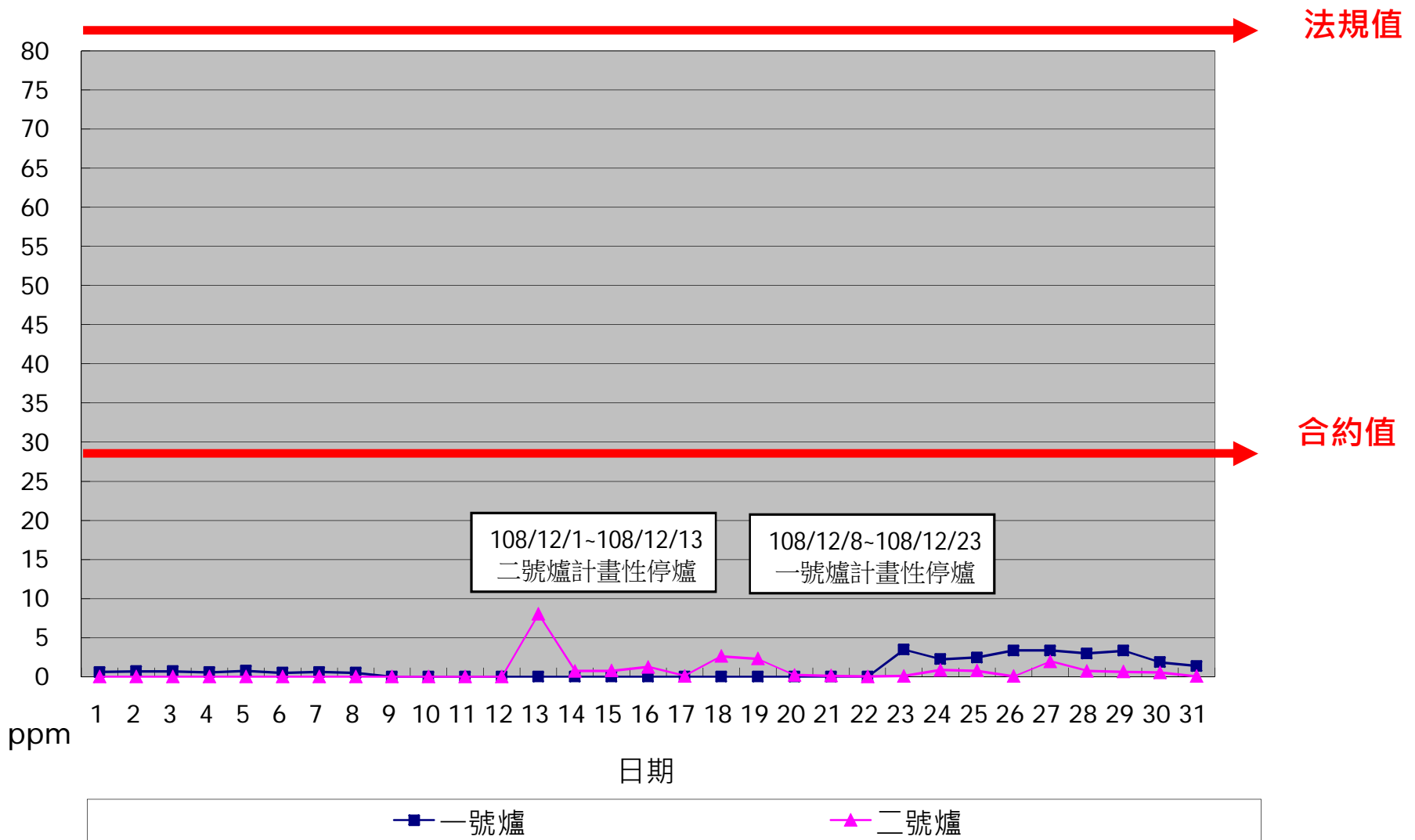
一百零八年十二月份 SO x 單日24小時整月排放監測紀錄
