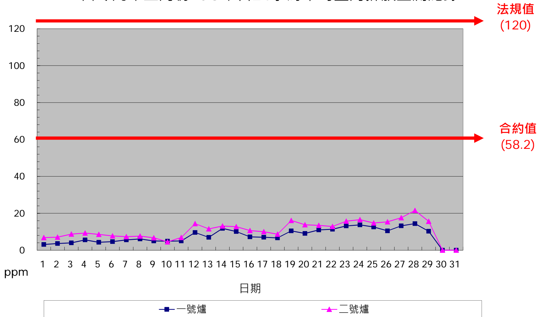
一百零九年二月份 CO 單日24小時平均整月排放監測紀錄
