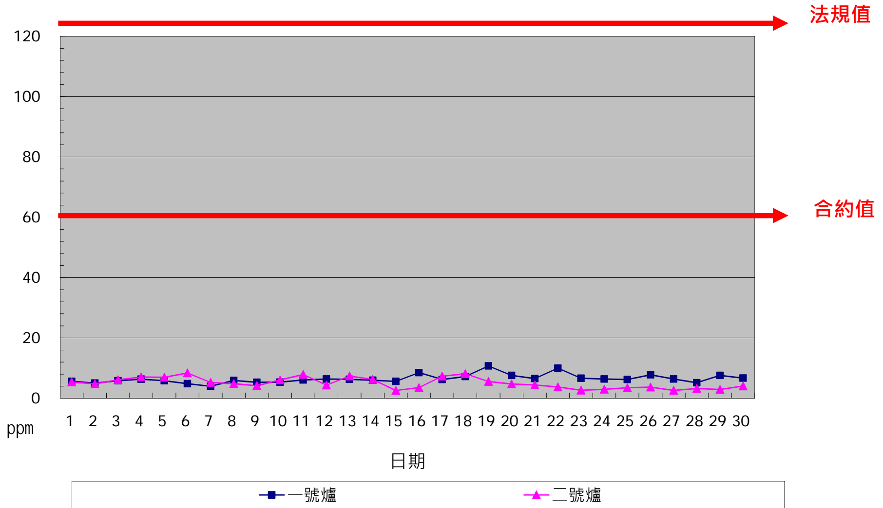
一百零九年六月份 CO單日24小時平均整月排放監測紀錄
