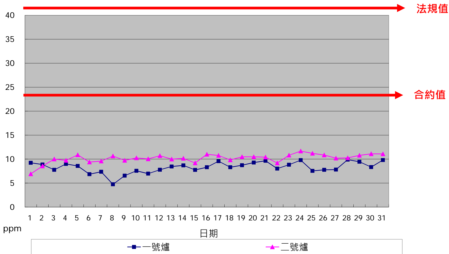
一百零九年七月份 HCl 單日24小時整月排放監測紀錄
