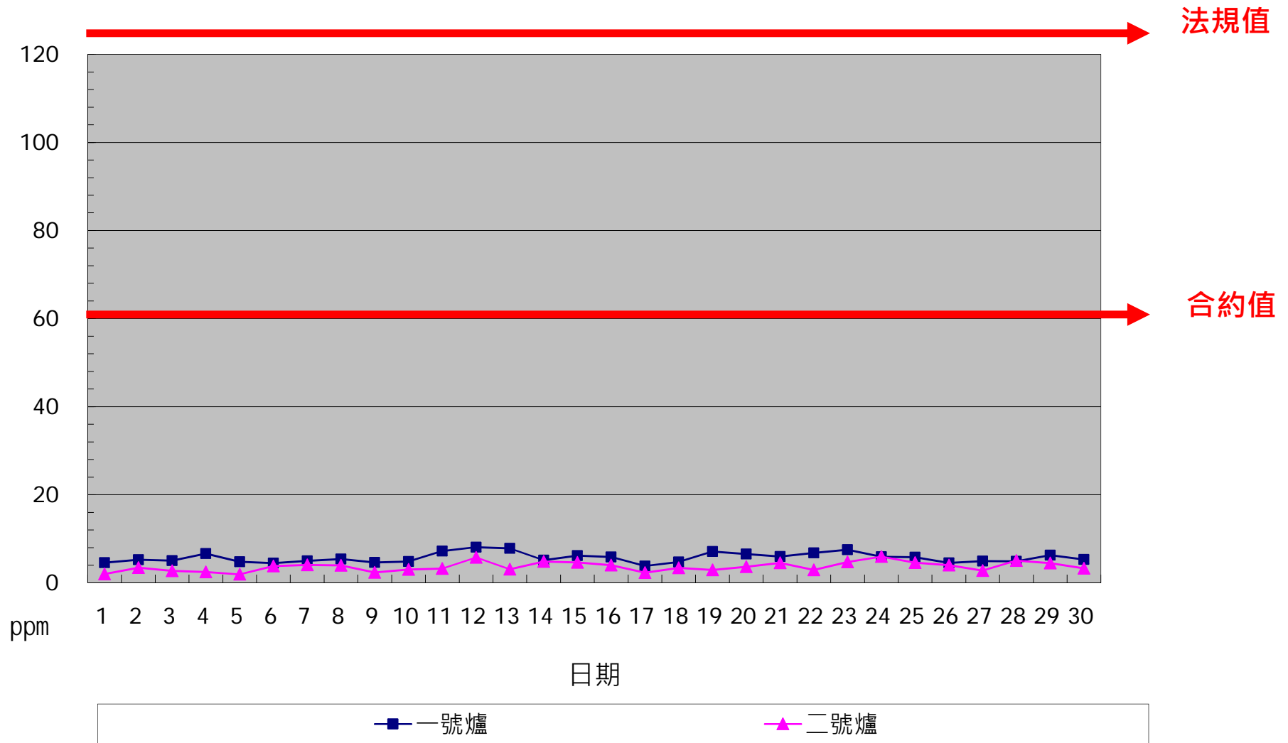
一百零九年九月份 CO單日24小時平均整月排放監測紀錄
