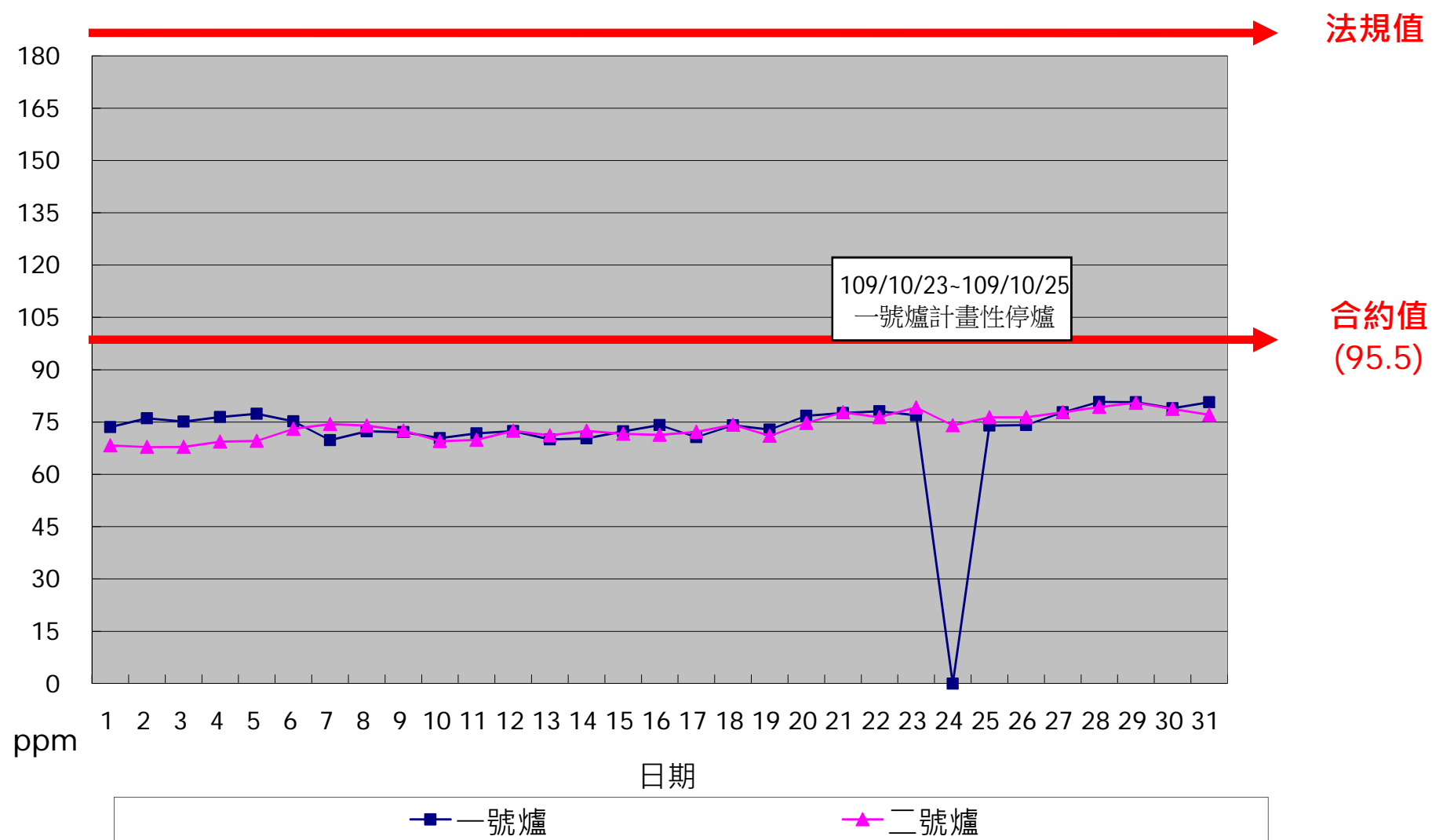
一百零九年十月份 NO x 單日24小時整月排放監測紀錄
