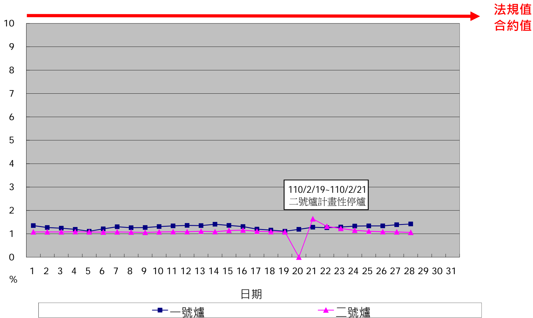
一百一十年二月份 OPACITY單日24小時整月排放監測紀錄
