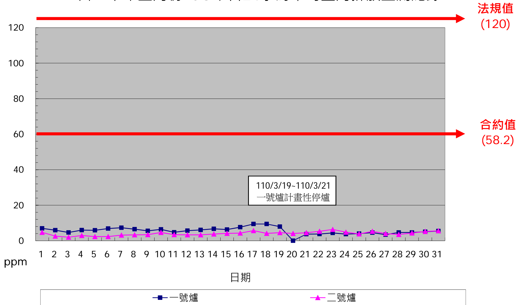
一百一十年三月份 CO 單日24小時平均整月排放監測紀錄
