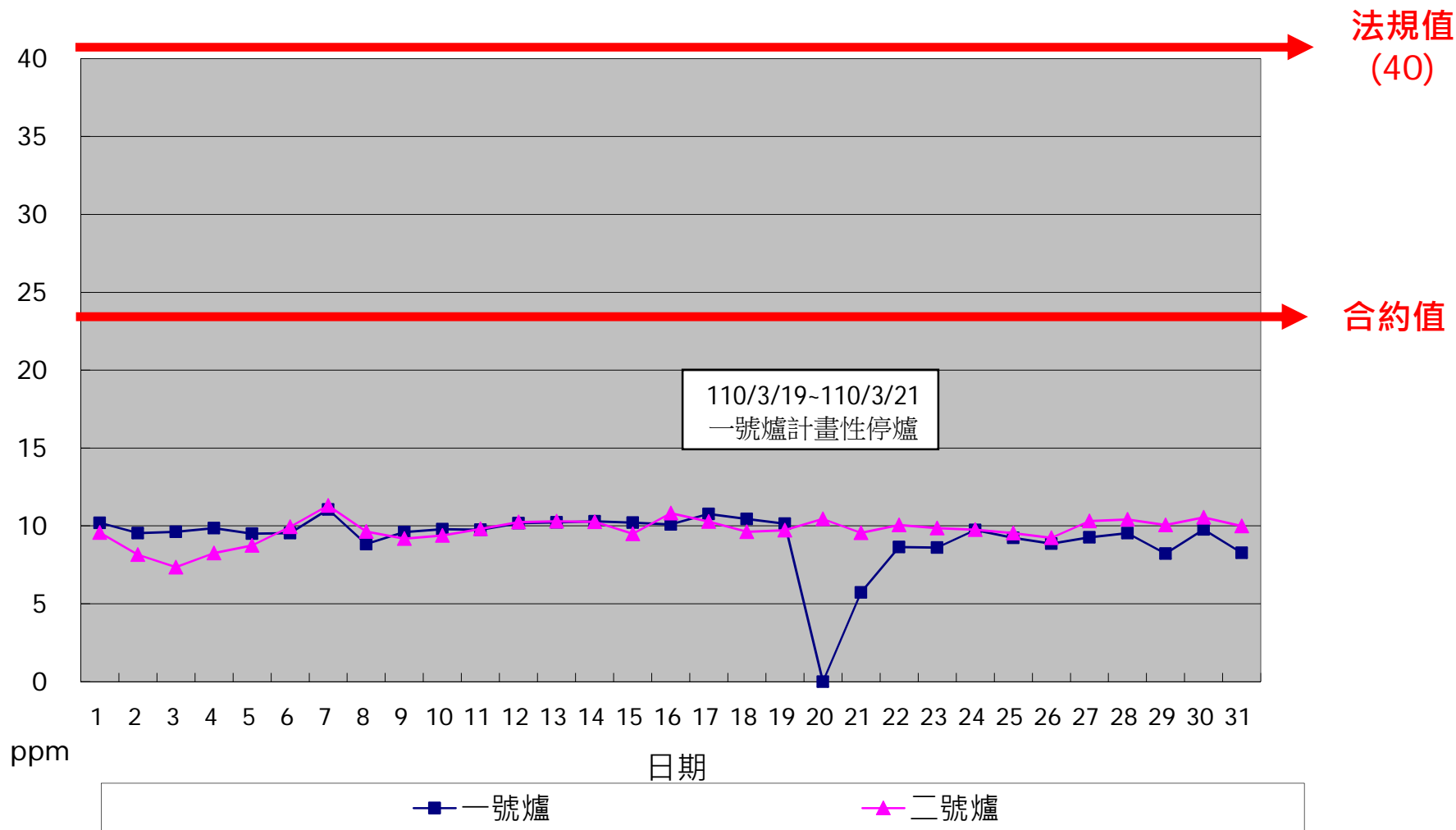
一百一十年三月份 HCl 單日24小時整月排放監測紀錄
