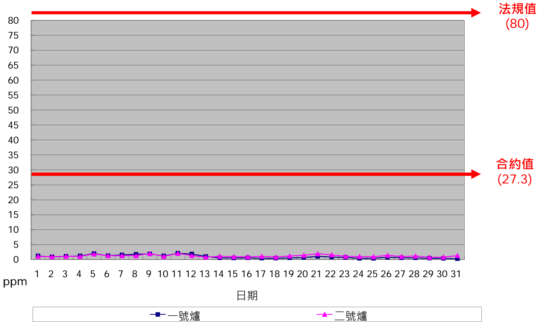
一百一十年七月份 SO x 單日24小時整月排放監測紀錄
